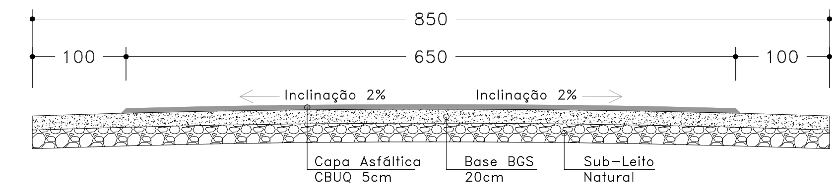
CORTE - Construção da pista
