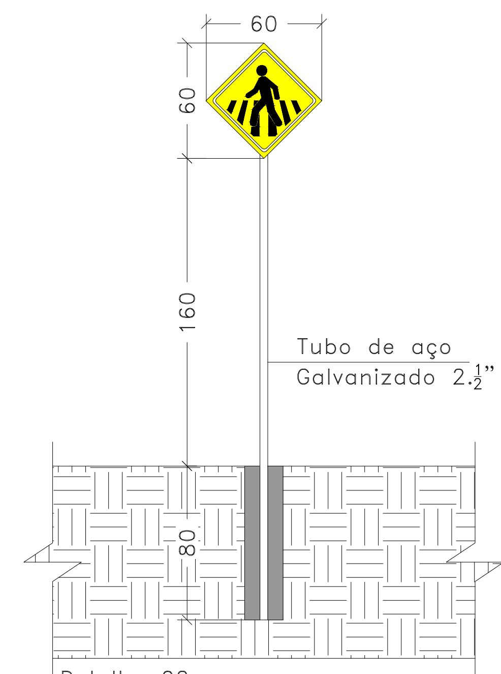
Detalhe 02 Sinalização Viária Vertical
