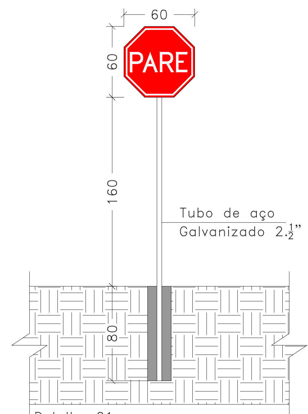
Detalhe 01 Sinalização Viária Vertical
